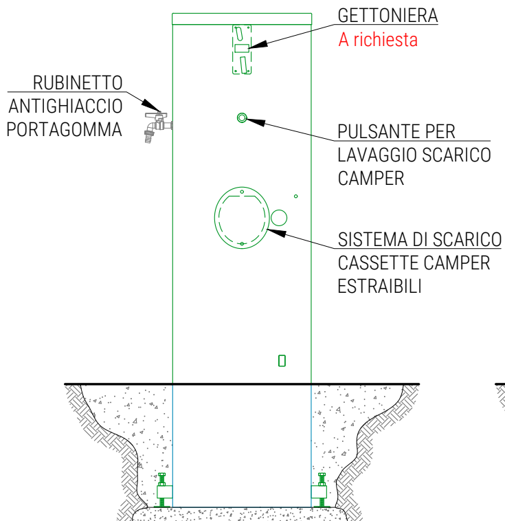
FRONTE
