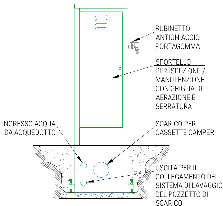
RETRO
