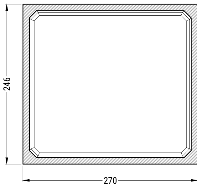
PIANTA VASCA
