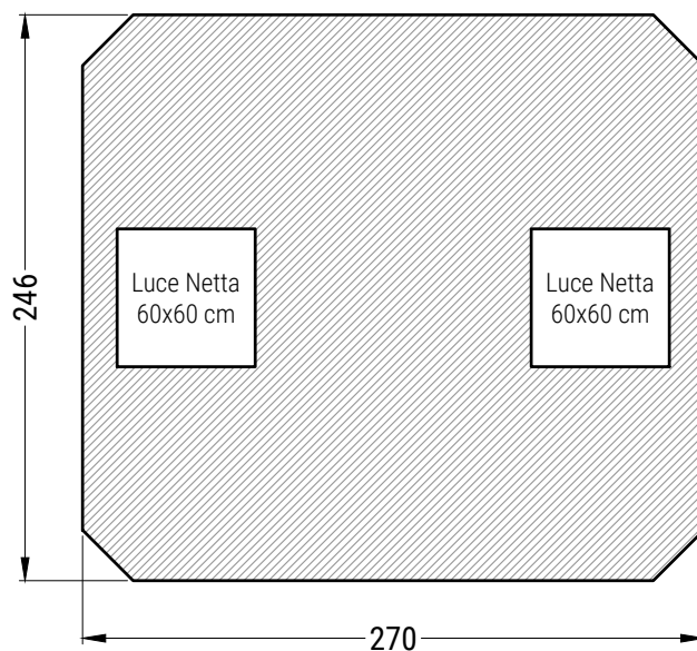
PIANTA COPERTURA
