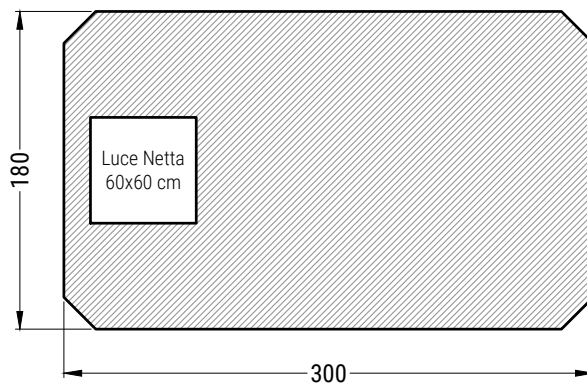
PIANTA COPERTURA
