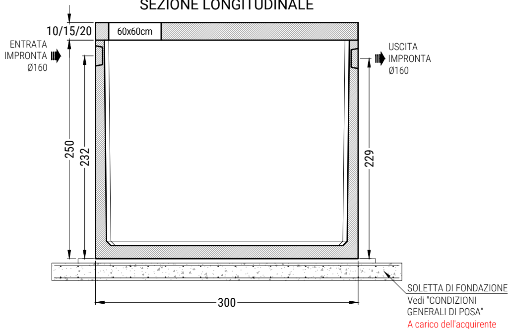
SEZIONE LONGITUDINALE
