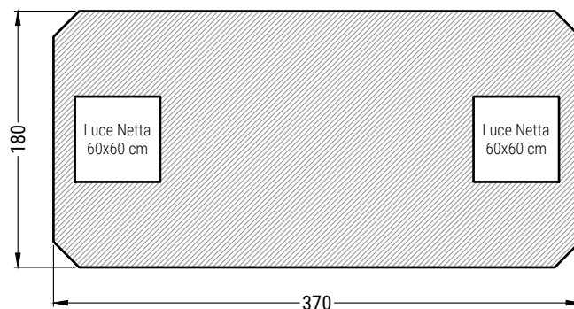
PIANTA COPERTURA
