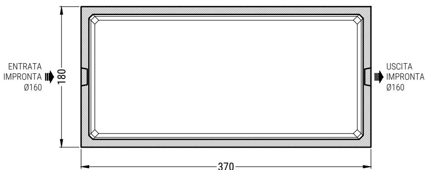
PIANTA COPERTURA
