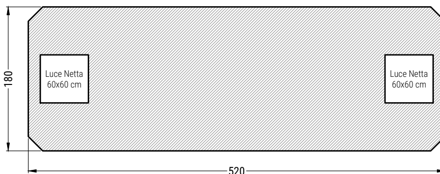
PIANTA COPERTURA
