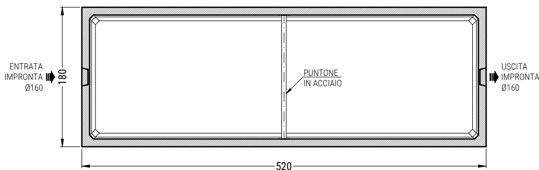
PIANTA COPERTURA
