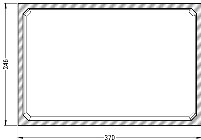
PIANTA VASCA
