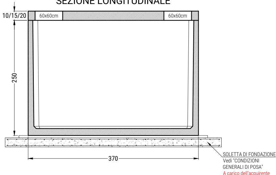
SEZIONE LONGITUDINALE
