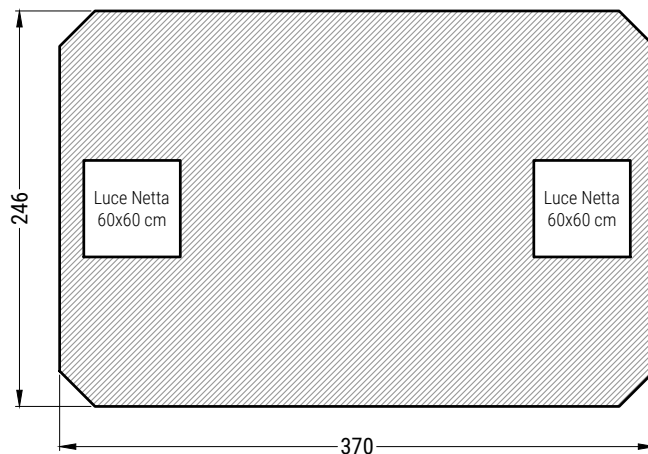
PIANTA COPERTURA
