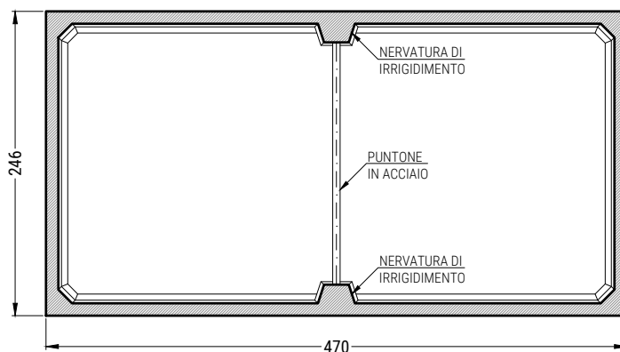
PIANTA COPERTURA
