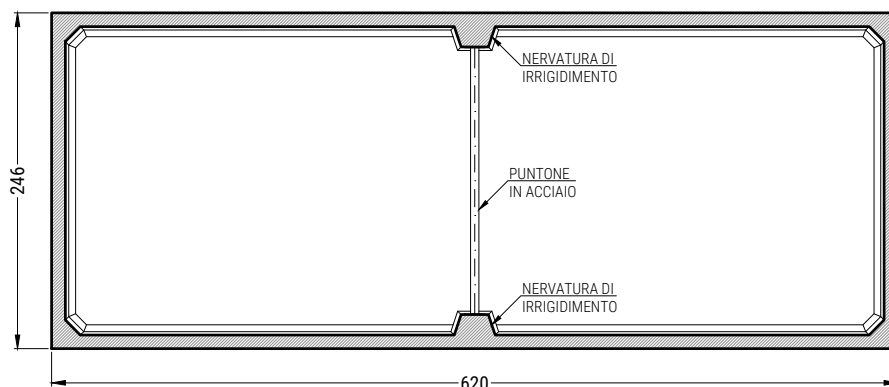
PIANTA COPERTURA
