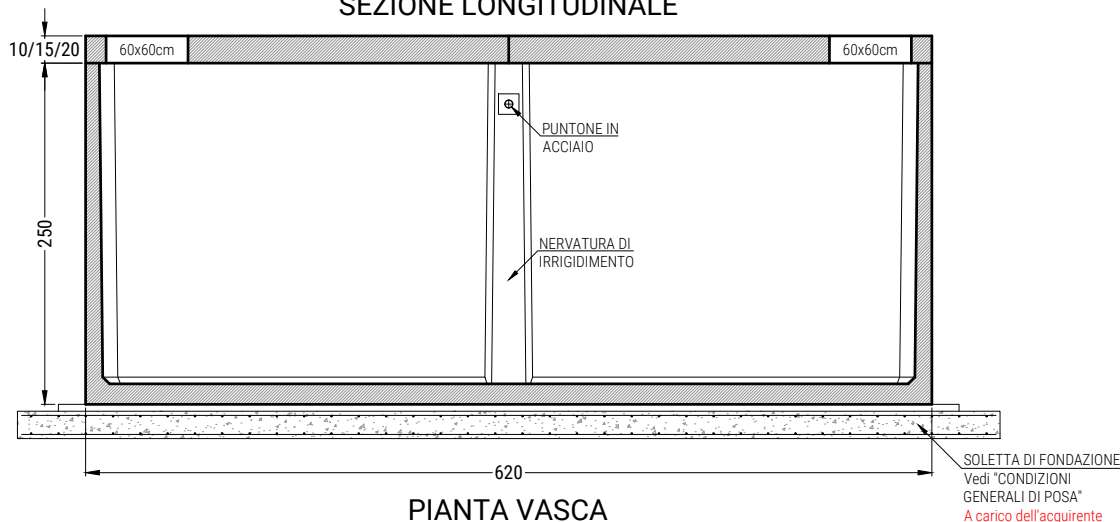
SEZIONE LONGITUDINALE
