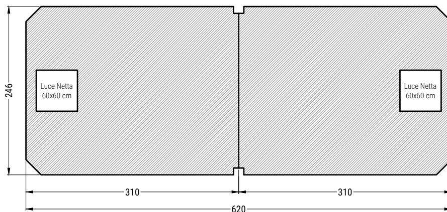
PIANTA COPERTURA
