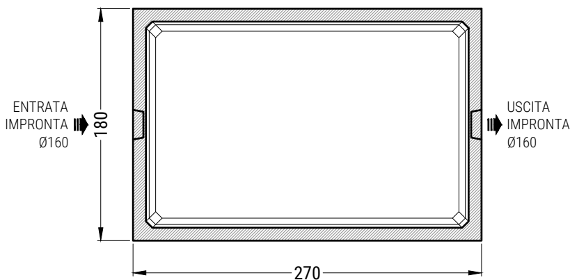
PIANTA VASCA
