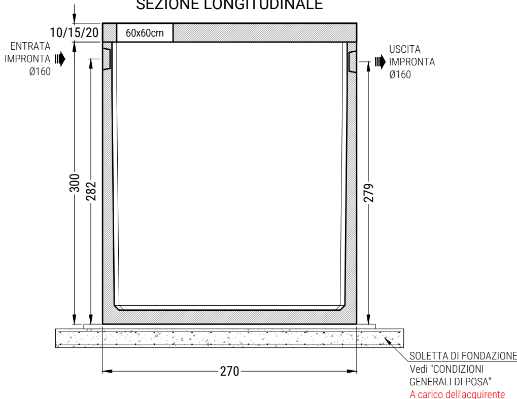
SEZIONE LONGITUDINALE
