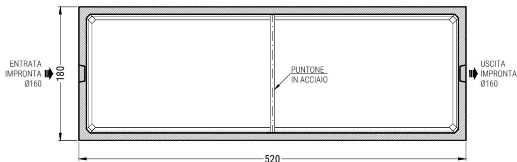
PIANTA COPERTURA
