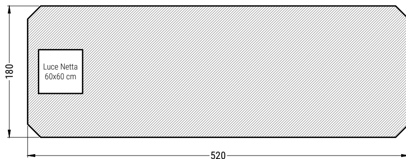
PIANTA COPERTURA
