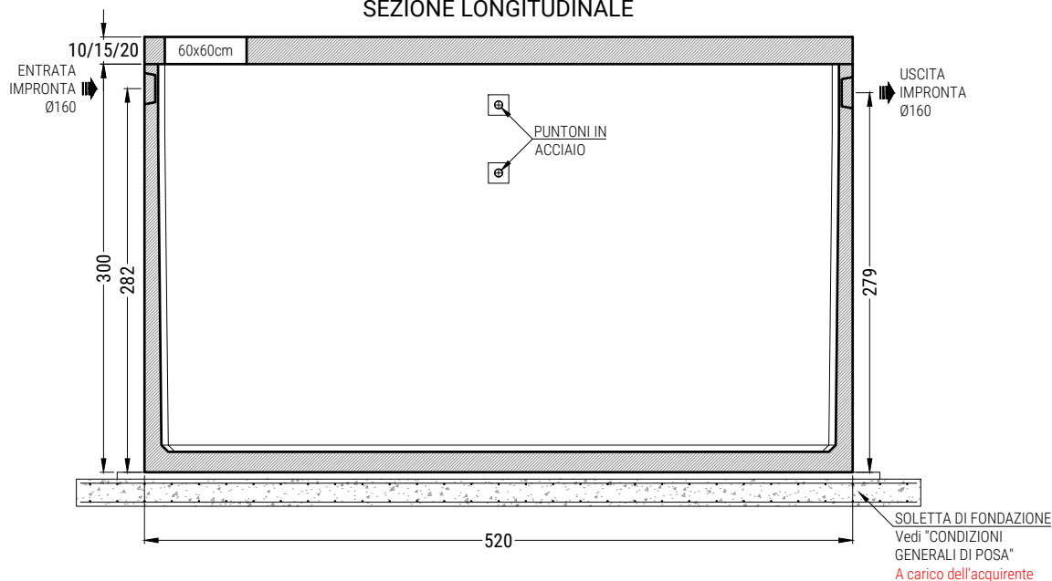
PIANTA VASCA
