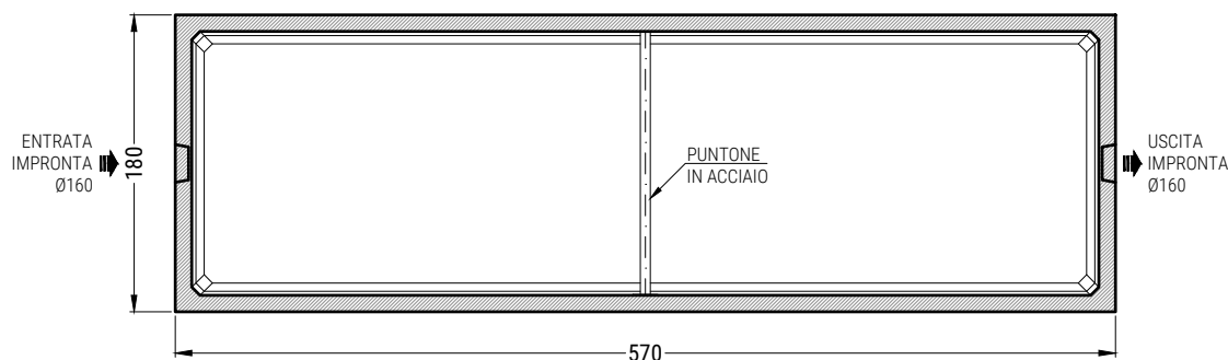
PIANTA COPERTURA
