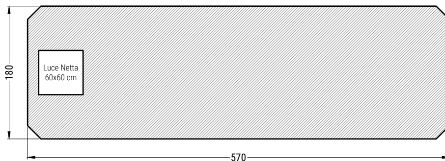
PIANTA COPERTURA
