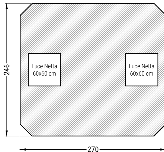
PIANTA COPERTURA
