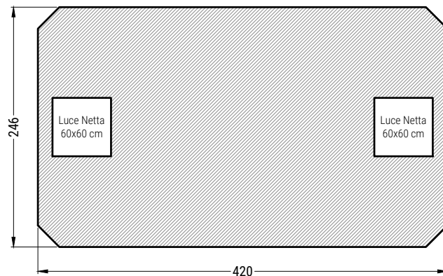
PIANTA COPERTURA
