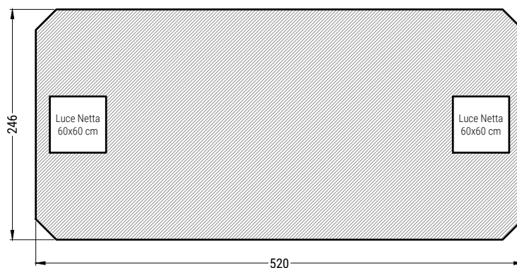
PIANTA COPERTURA
