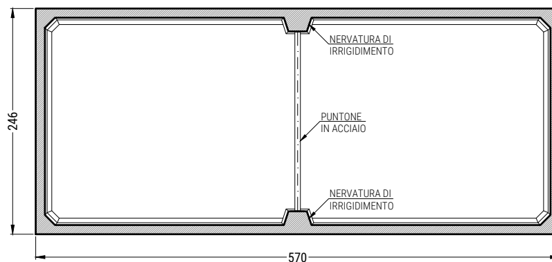
PIANTA COPERTURA
