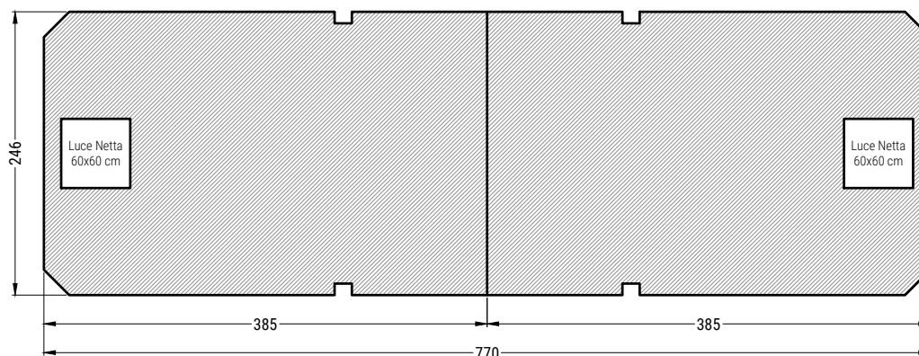
PIANTA COPERTURA
