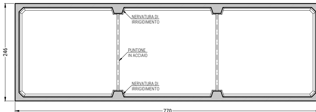
PIANTA COPERTURA
