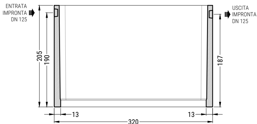
SEZIONE LONGITUDINALE
