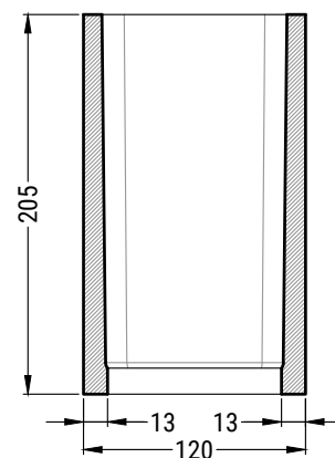
SEZIONE TRASVERSALE
