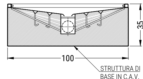
SEZIONE TRASVERSALE
