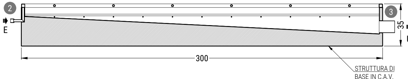
SEZIONE LONGITUDINALE
