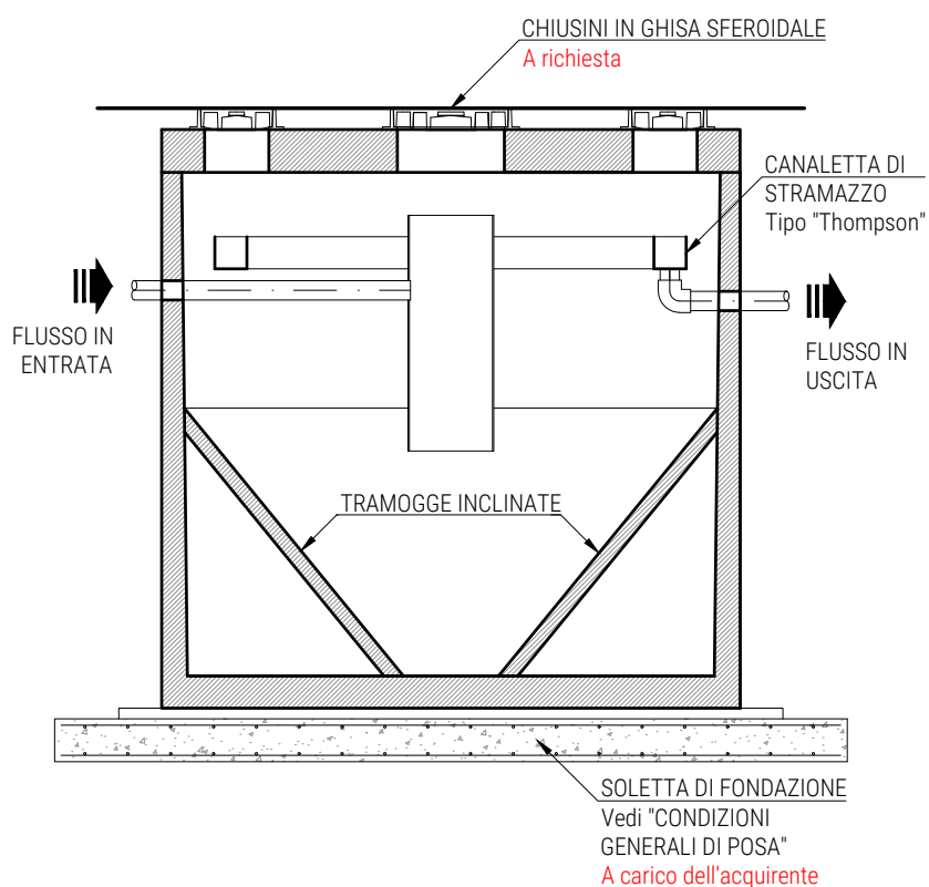
SEZIONE LONGITUDINALE
