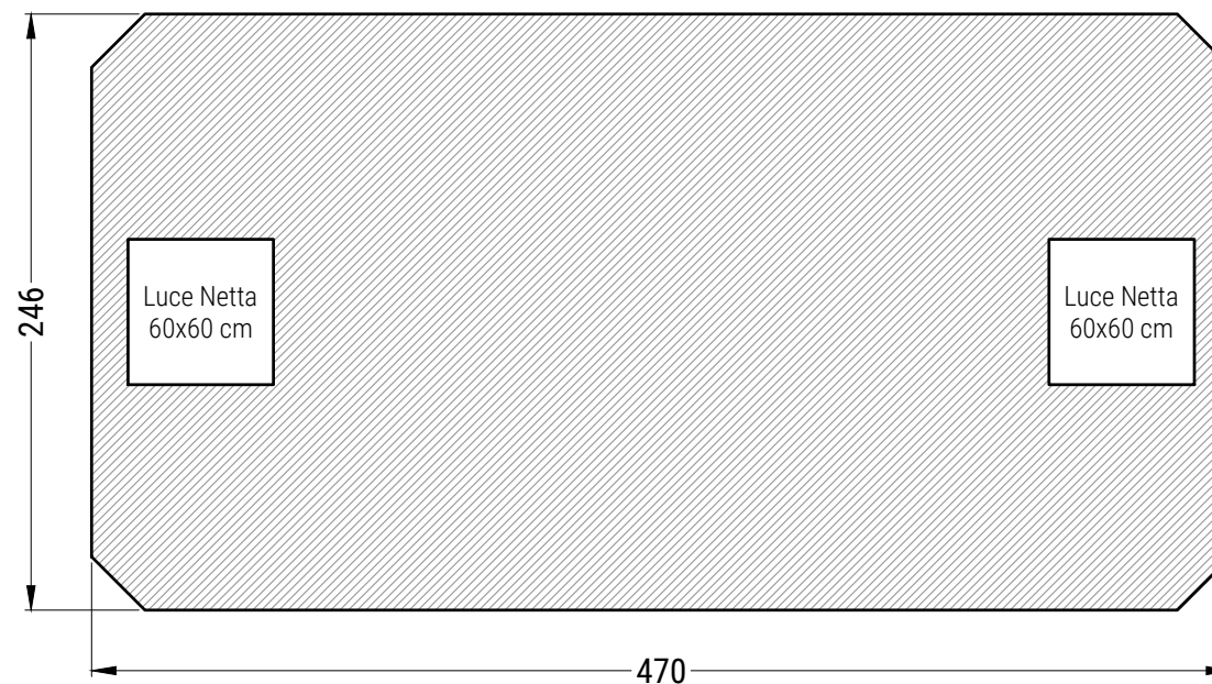
PIANTA COPERTURA
