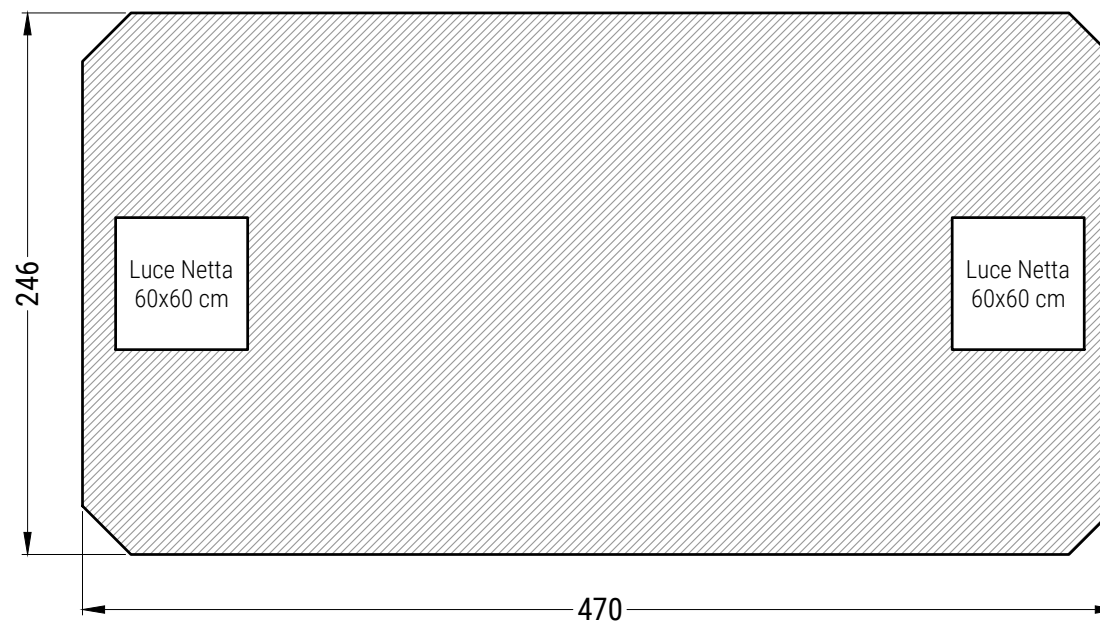
PIANTA COPERTURA
